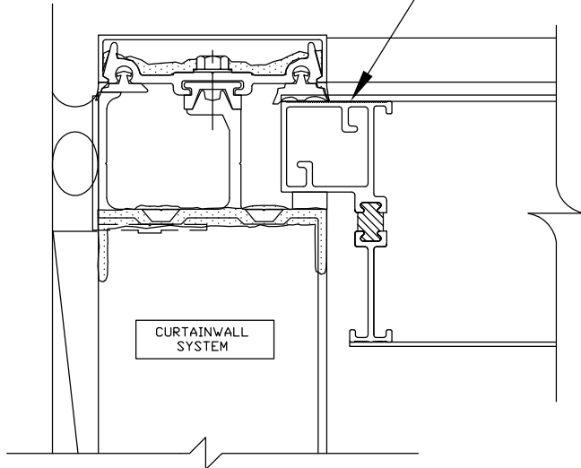
JAMB DETAIL
