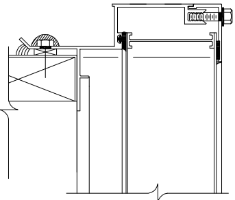
3 1 - - JAMB DETAIL
